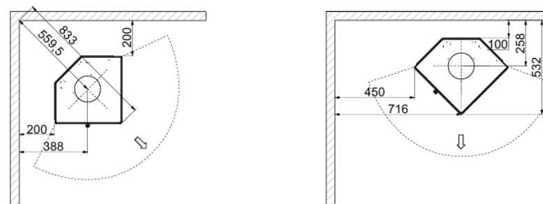
Mindestabstände zu brennbaren Materialien
