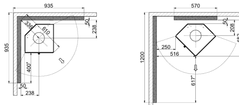
Mindestabstände zu brennbaren Materialien
