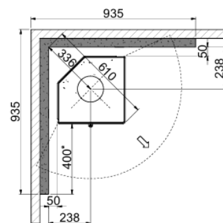
Mindestabstände zur brennbaren Wand, geschützt mit Brandschutzwand
