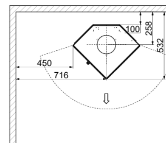
Mindestabstände zu brennbaren Materialien
