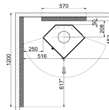
Mindestabstände zu brennbaren Materialien
